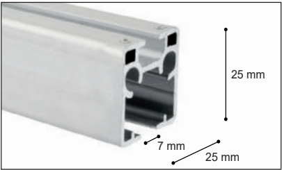
Perfil Sintra® (Cordón y Manual)
