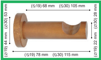
Soporte Madera Cilindro
