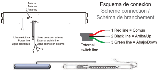
Esquema de conexión Batería Externa
