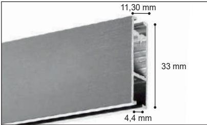
Perfil Aluminio
