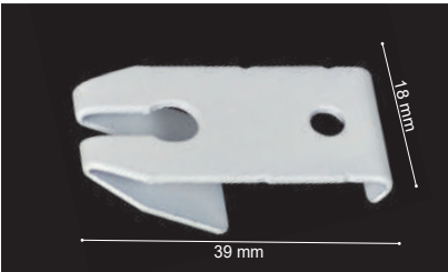
Soporte techo Abierto Invisible Invisible Open Ceiling Bracket / Support Plafond Ouvert Invisible
