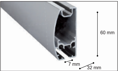
Perfiles Coimbra® (Cordón y Manual)
