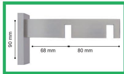
Soporte Doble Pared
