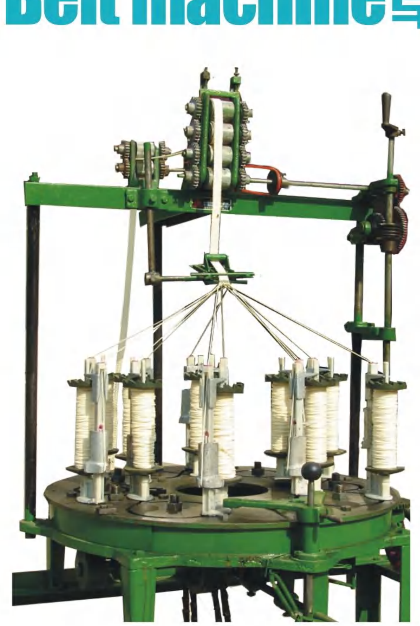
Flat11 扁11锭草编机
