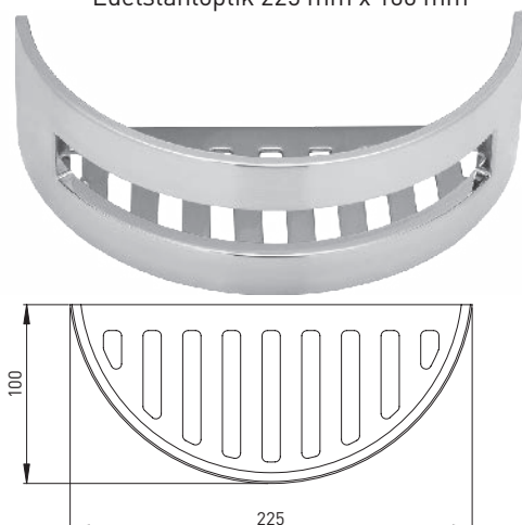
104638 Schwammkorb geschlossen komplett mit Befestigung Edelstahloptik 225 mm x 100 mm
