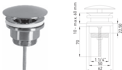
106442 Design-Universalventil 1 1/4" x Ø 63 mm Stopfen Ø 72 mm, rund, Messing Edelstahloptik, nicht verschließbar
