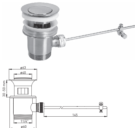
100447 Excentergarnitur 1 1/4" x Ø 63 mm mit Excenterstopfen Standard Ø 40 mm mit Überlaufschlitzen Messing Edelstahloptik
