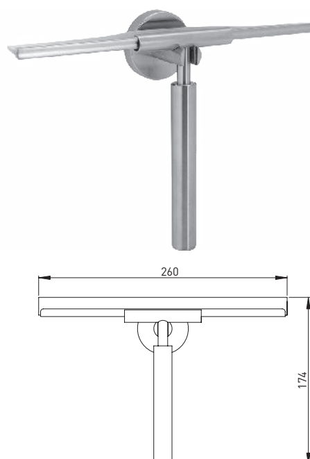
213772 Glasreiniger mit Wandhalterung Messing Edelstahloptik
