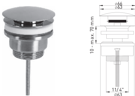
106723 Design-Universalventil 1 1/4" x Ø 63 mm Stopfen Ø 66 mm, rund, Messing Edelstahloptik, verschließbar
