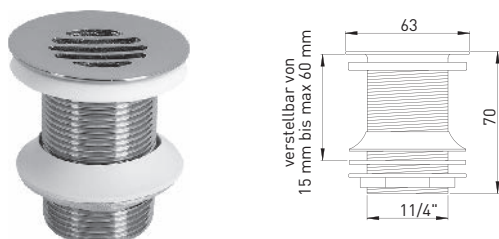
107691 Schaftventil 1 1/4" x Ø 63 mm mit Siebeinlauf, ohne Überlaufschlitze Schaftlänge: 70 mm, Messing Edelstahloptik
