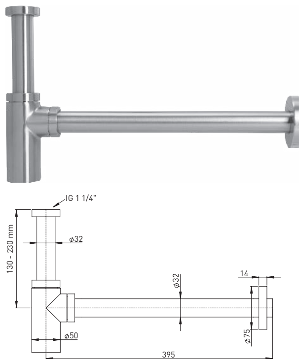
110131 Design-Geruchverschluss "PLUS" 1 1/4" x 32 mm Verstellrohr 200 mm, Rosette 75 mm Wandrohr 370 mm, verschraubt Messing Edelstahloptik
