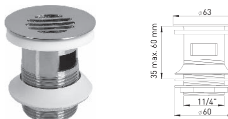
100400 Schaftventil 1 1/4" x Ø 63 mm mit Siebeinlauf, mit Überlaufschlitzen Schaftlänge: 70 mm, Messing Edelstahloptik
