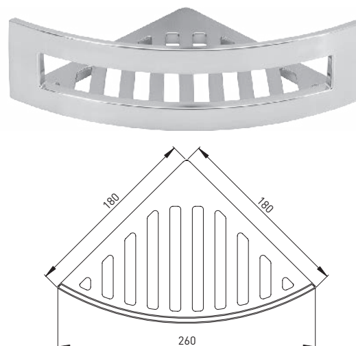
104664 Eckschwammkorb geschlossen komplett mit Befestigung Edelstahloptik 260 mm x 180 mm
