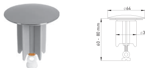
100417 Excenterstopfen Universal 1 1/4" Platte Ø 64 mm, passend für alle Fabrikate Dichtung weiß, Messing Edelstahloptik
