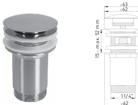
105748 Design-Abflussventil 1 1/4" x Ø 63 mm Stopfen Ø 62 mm Messing Edelstahloptik mit Überlaufschlitzen, verschließbar
