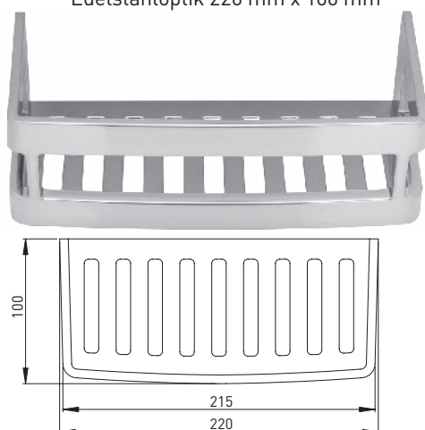
104612 Schwammkorb geschlossen komplett mit Befestigung Edelstahloptik 220 mm x 100 mm
