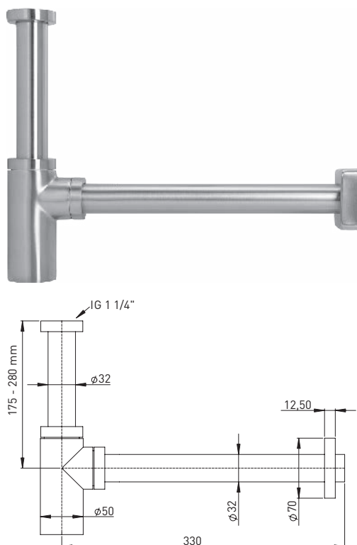
110736 Design Geruchverschluss 1 1/4" x 32 mm je 1 runde (Ø 70 mm) und eckige (64x64 mm) Rosette Verstellrohr 250 mm, Wandrohr 300 mm Messing Edelstahloptik
