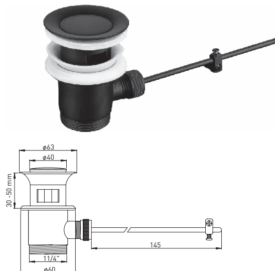
102605 Excentergarnitur 1 1/4" x Ø 63 mm mit Excenterstopfen Standard Ø 40 mm mit Überlaufschlitzen Messing matt schwarz
