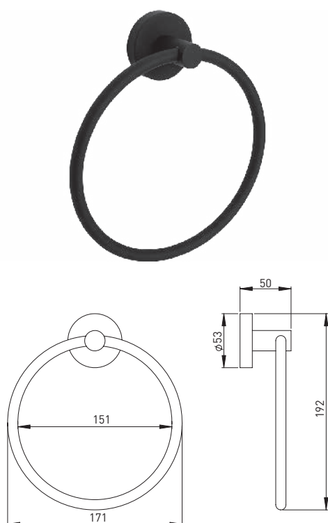
211561 Handtuchring Messing matt schwarz
