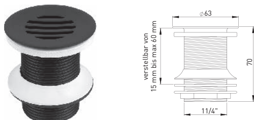
107663 Schaftventil 1 1/4" x Ø 63 mm mit Siebeinlauf, ohne Überlaufschlitze Schaftlänge: 70 mm, Messing matt schwarz
