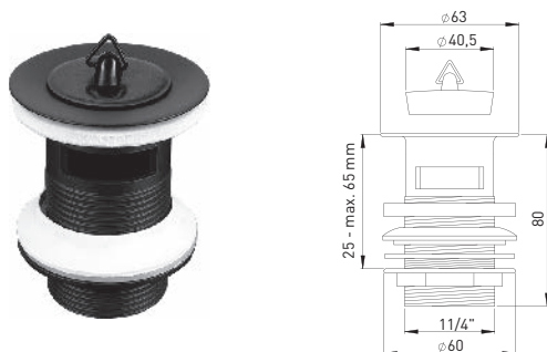
108392 Schaftventil 1 1/4" x Ø 63 mm mit Überlaufschlitzen und Stopfen Schaftlänge 80 mm, Messing matt schwarz
