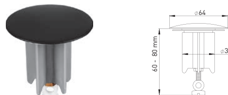
102533 Excenterstopfen Universal 1 1/4" Platte Ø 64 mm, passend für alle Fabrikate Dichtung weiß, Messing matt schwarz
