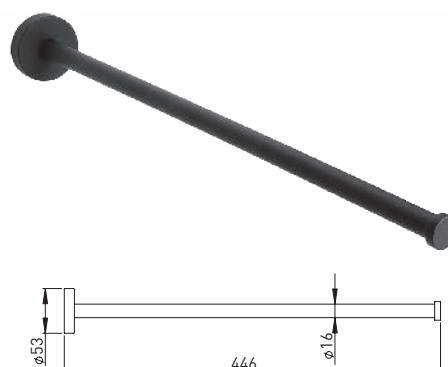
211518 Handtuchhalter 1-armig Messing matt schwarz
