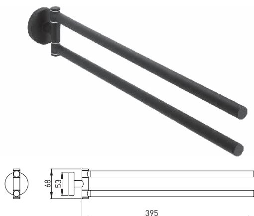
211445 Handtuchhalter 2-armig Messing matt schwarz
