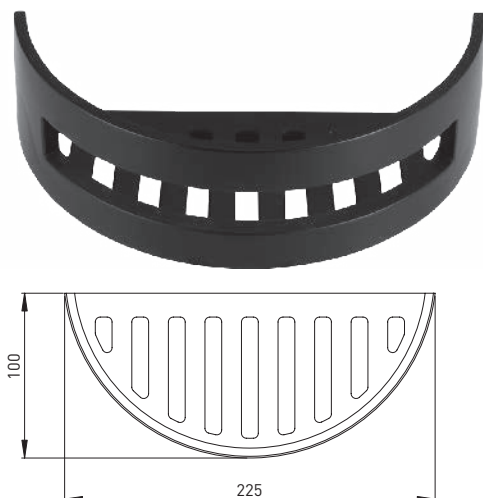
104599 Schwammkorb geschlossen komplett mit Befestigung matt schwarz 225 mm x 100 mm
