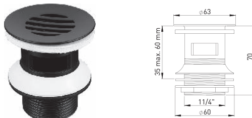
108462 Schaftventil 1 1/4" x Ø 63 mm mit Siebeinlauf, mit Überlaufschlitzen Schaftlänge: 70 mm, Messing matt schwarz
